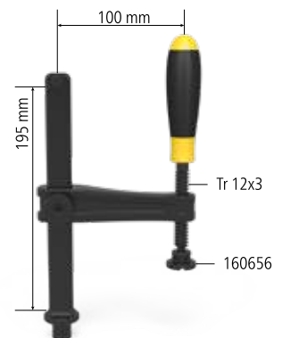
2-160620 Morsetto a vite Basic - brunito 59,00 € •
