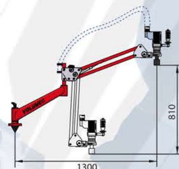
DOPPIO BRACCIO ARTICOLATO JT2 RAGGIO DI LAVORO 1300 mm
